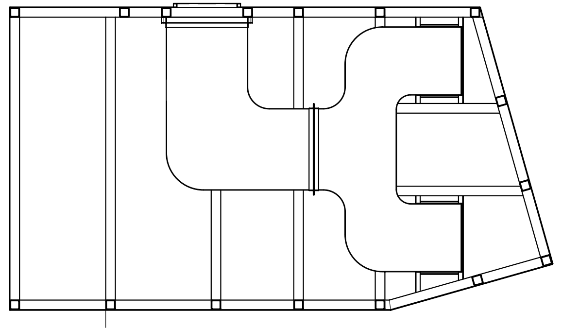
F-F(风管安装示意图) Схема монтажа воздуховода
